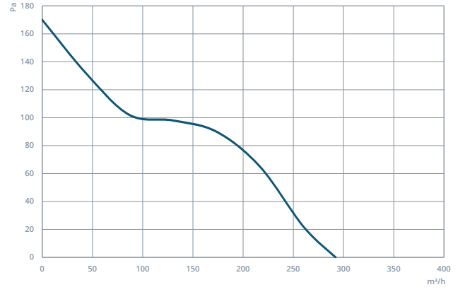
KAP 125
