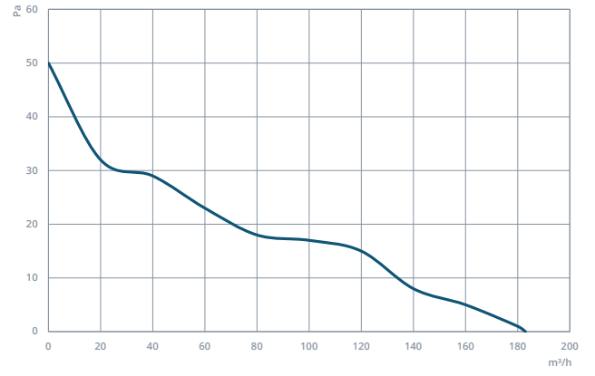
BAF 125
