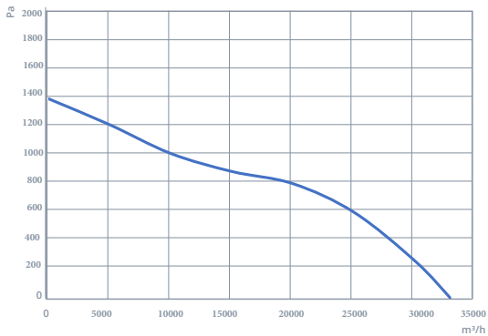
AXI 630-8-45
