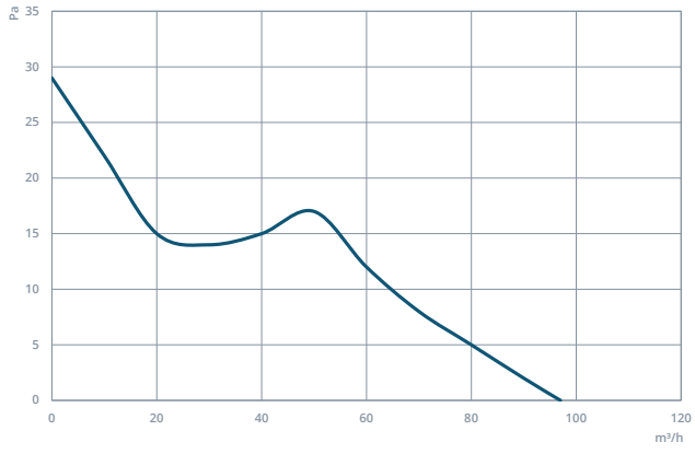
BAF 100
