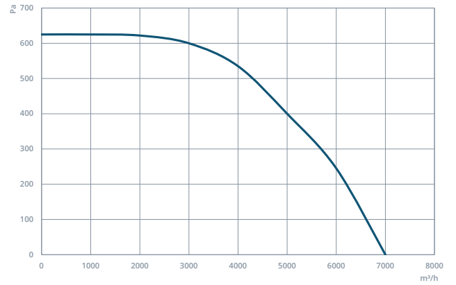
DRAD 500
