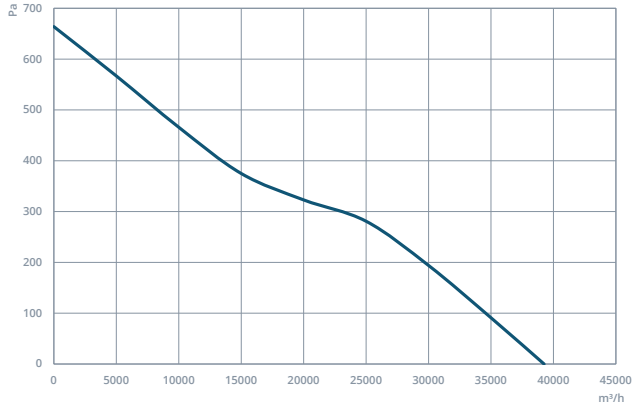
HAXI 900-5-35
