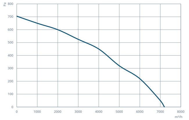
KASP 560
