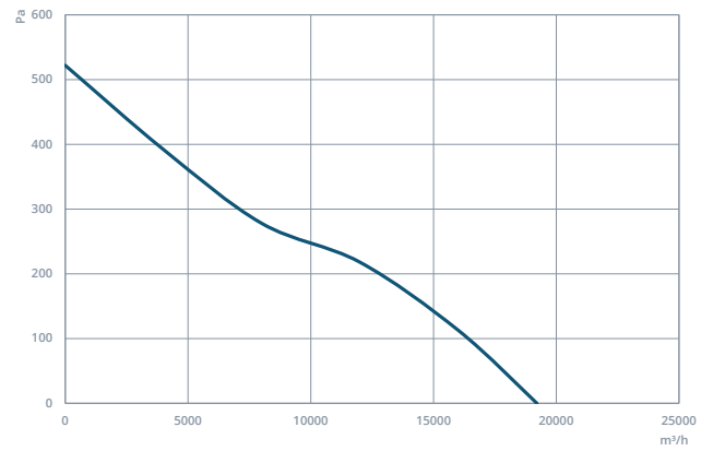
HAXI 710-5-30
