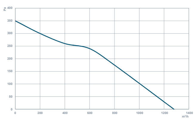
KAF 250
