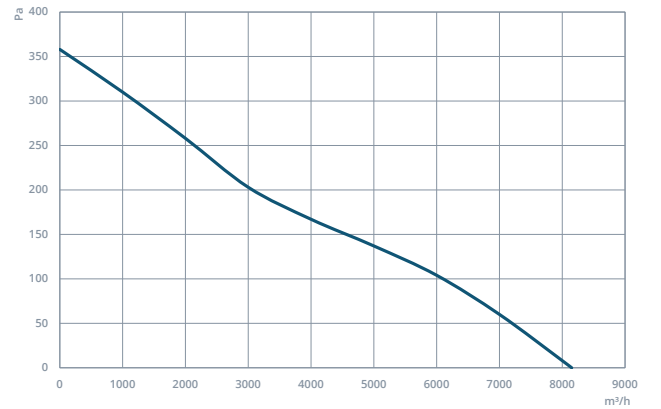
AXIP 560-5-25
