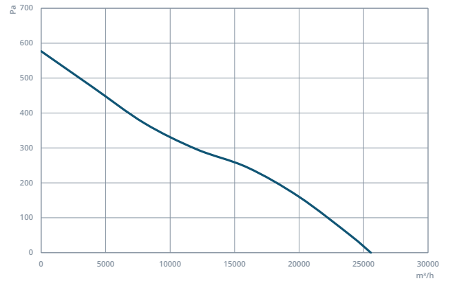
GAXI 800-5-30
