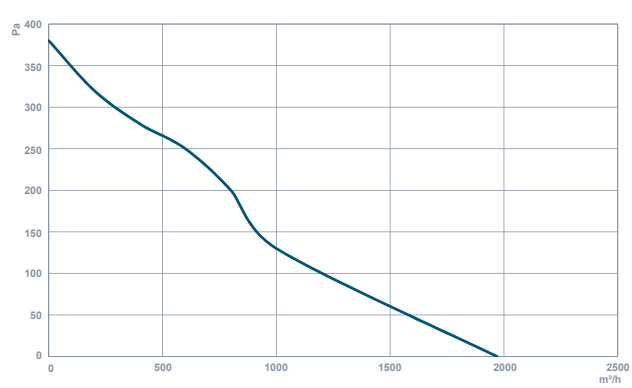
KAF 315
