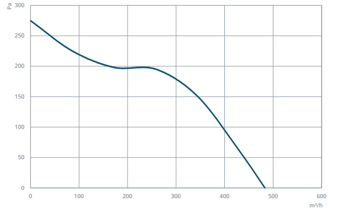
KAP 160
