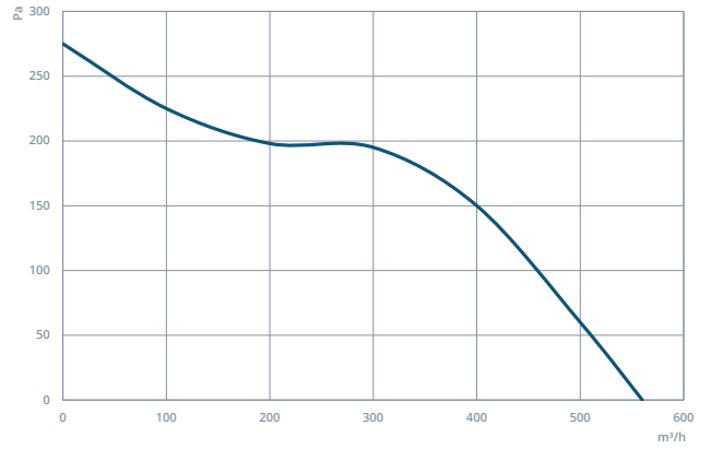
KAF 160
