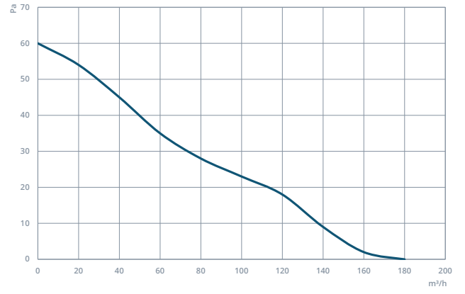
SEF 125
