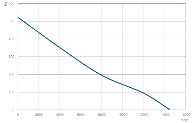
CAXIDIK 710-5-30
