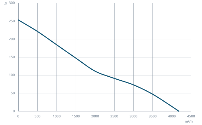
AXIP 450-5-25
