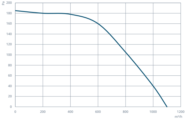
DRADIK 280
