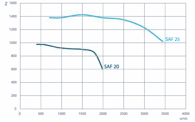
SAF 20-25
